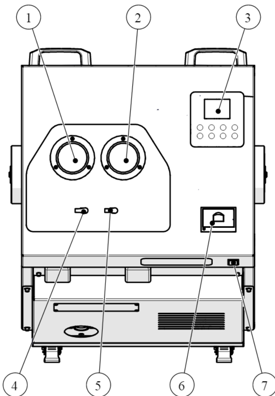
Рис. 3 Лицевая панель станции ODA-360A
