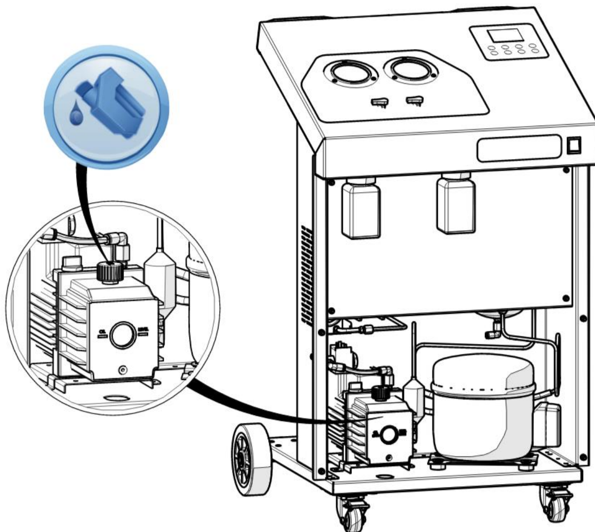
Рис. 9 Заправка вакуумного насоса
