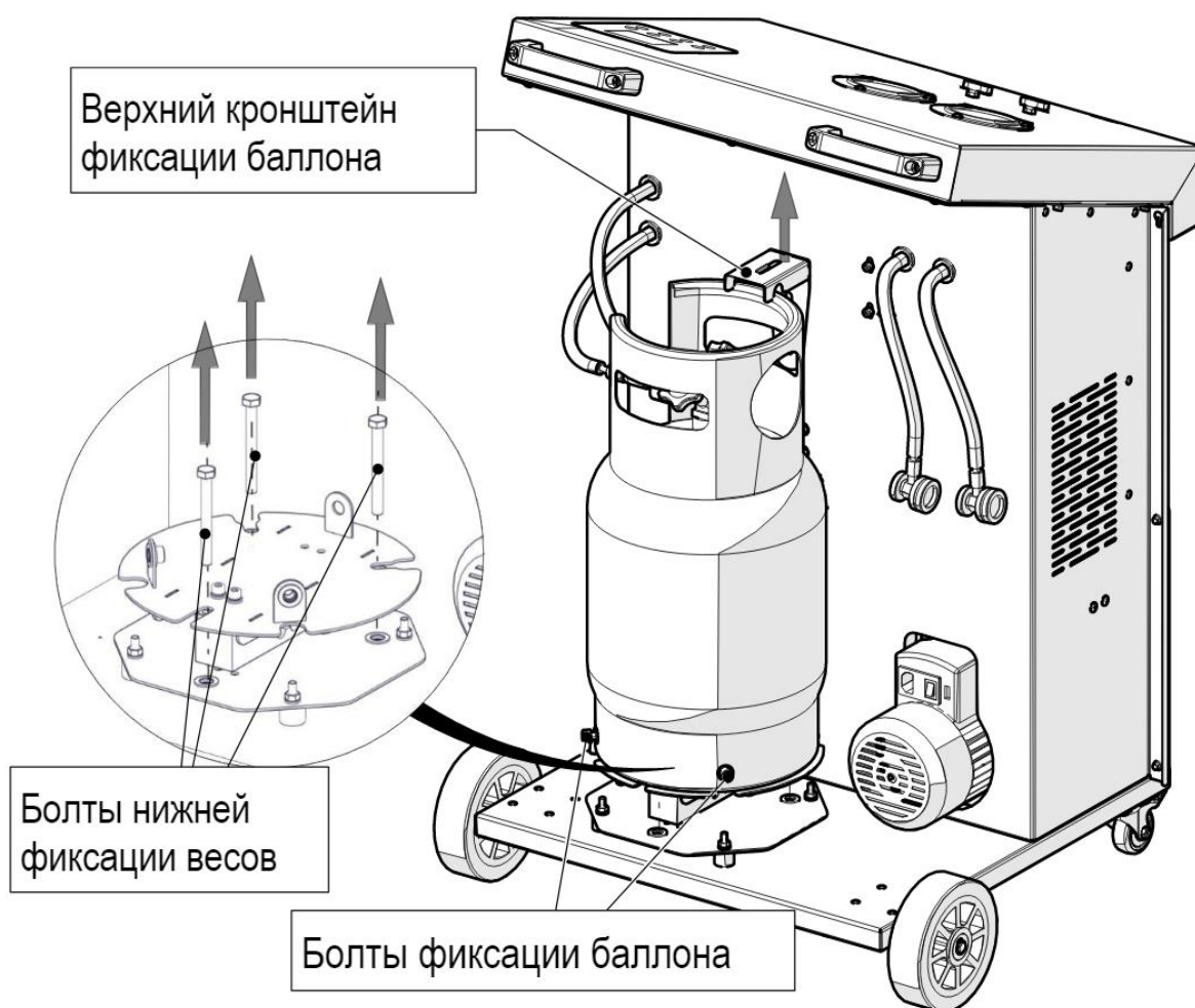
Рис. 5 Фиксация внутреннего баллона
