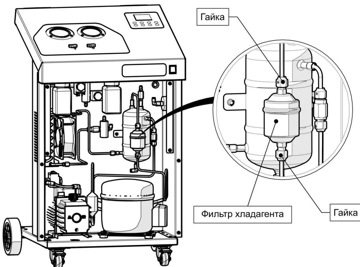
Рис. 10 Замена фильтра хладагента
