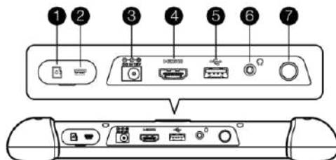
Рисунок 2-3 Диагностический сканер (вид сверху)
