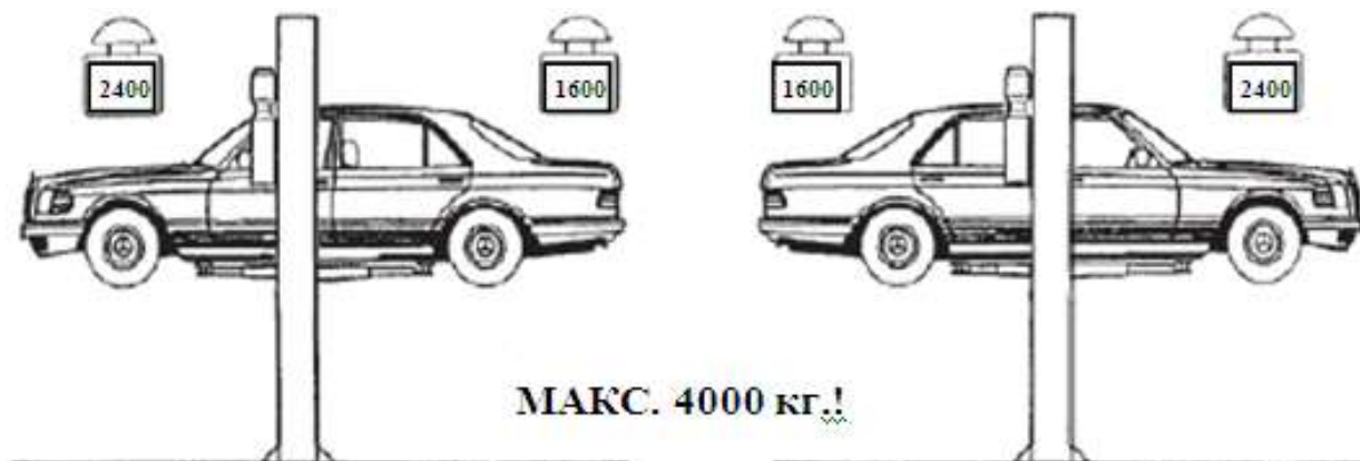
Рис. 10. Распределение веса.
