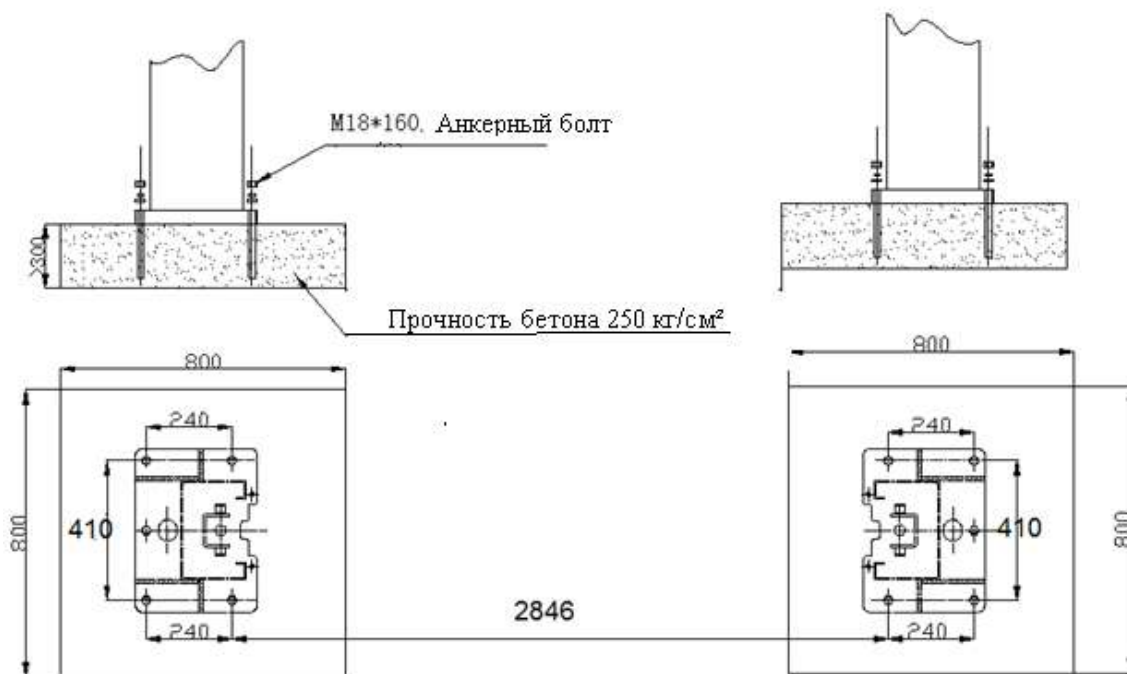
Рис. 1. Фундаментное задание.
